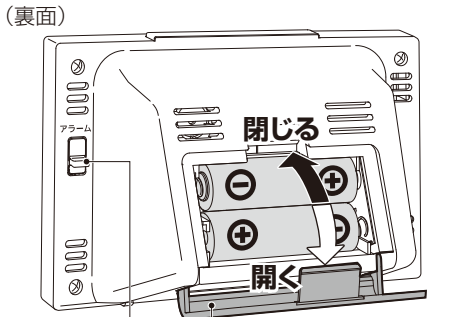
アラームスイッチ 電池ふた 単3形乾電池 2個
